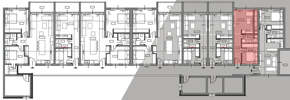
Kat daire yerleşimi
